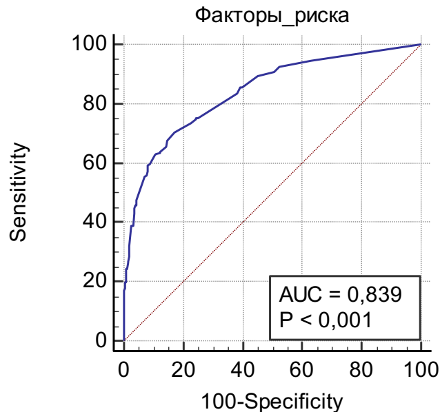
Рисунок 4 – ROC-кривая модели оценки ФР развития послеоперационных осложнений после маммопластики
